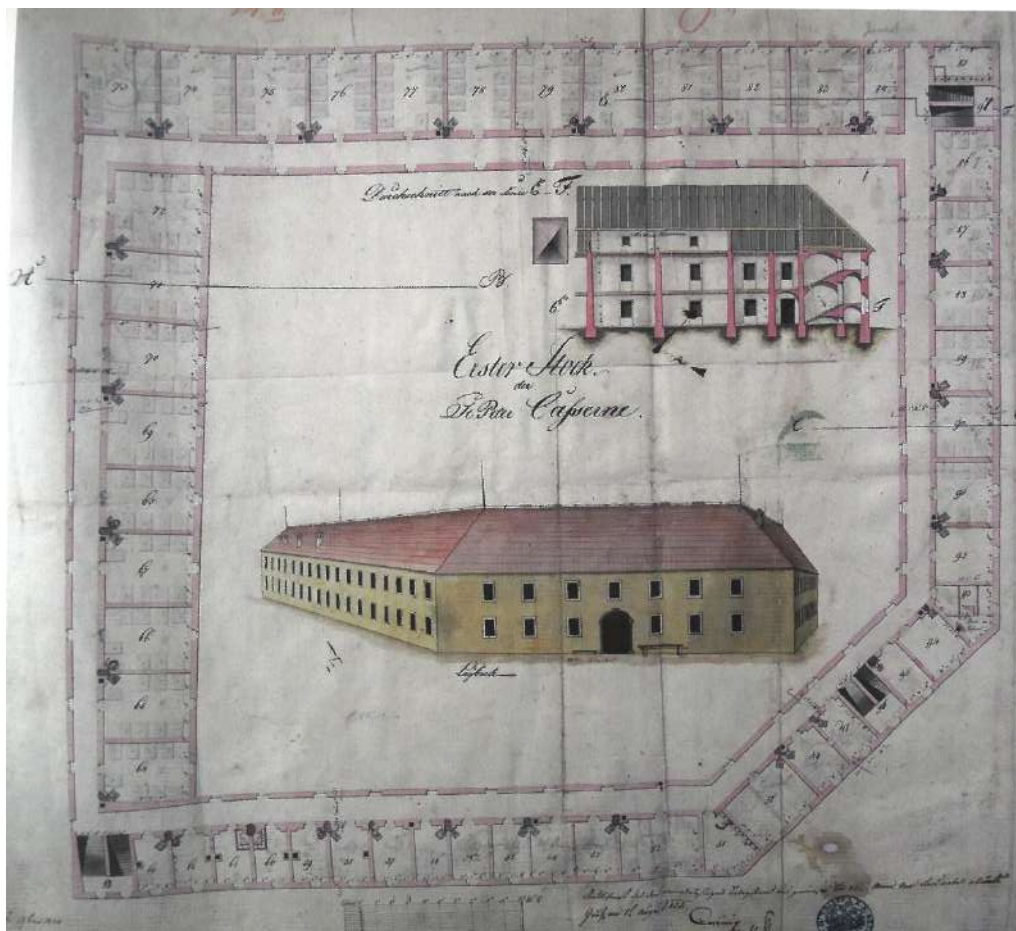
SLIKA 16: FASADA IN TLOVIS PRVEGA NADSTROPJA VOJAŠNICE V ŠENTPETRU PRI LJUBLJANI, RISBA, 1825 (OESTA KA, KPS GPA INLAND C III LAIBACH, ENVELOPE B, NR 1; FOTO: DUŠAN KOS)
